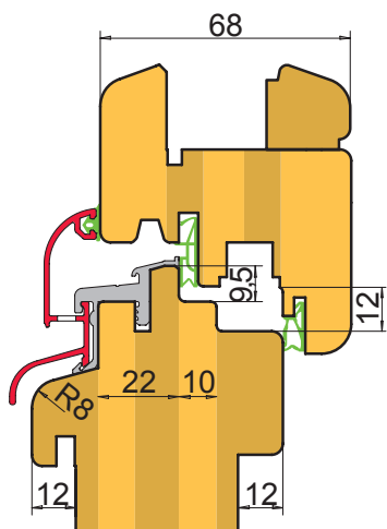
Šířka 68, kresleno s okapnicí MAIN 22/24 F-TI
