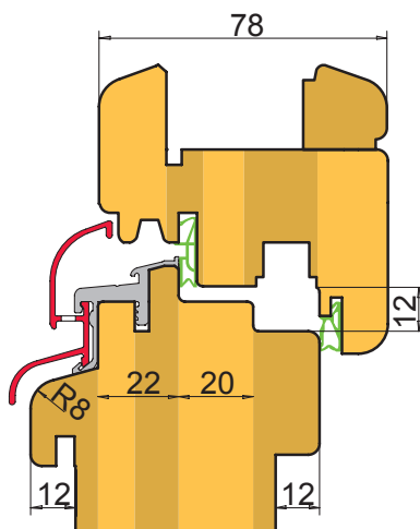
Šířka 78, kresleno s okapnicí DONAU 22/24 F-TI
