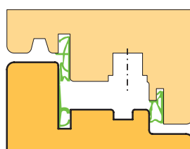
Šířka 78, kresleno s okapnicí DONAU 22/24 F-TI
