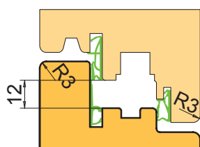
Šířka 68, kresleno s okapnicí MAIN 22/24 F-TI
