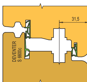
Kresleno s bezpečnostním kováním a oboustrannou dekompresní drážkou
