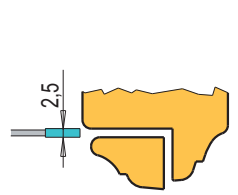
Odfíznutí lišty
