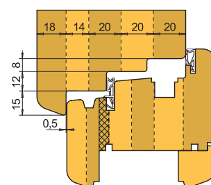
Pevné sady EURO 92 EURO 92 - trojitě těsnění
